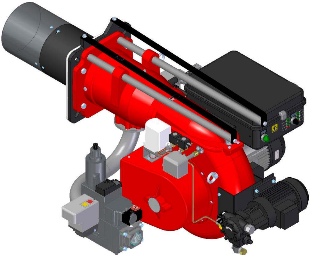
Fig. 1 MXP150/2
