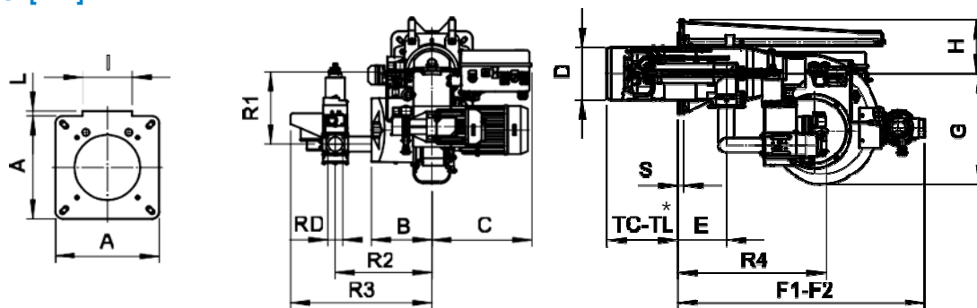
Fig. 3 Dimensions MXP 65/2 - 100/2 - 150/2
