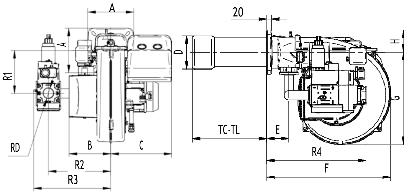
Fig. 3 Dimensions CXP45/2 MAX
