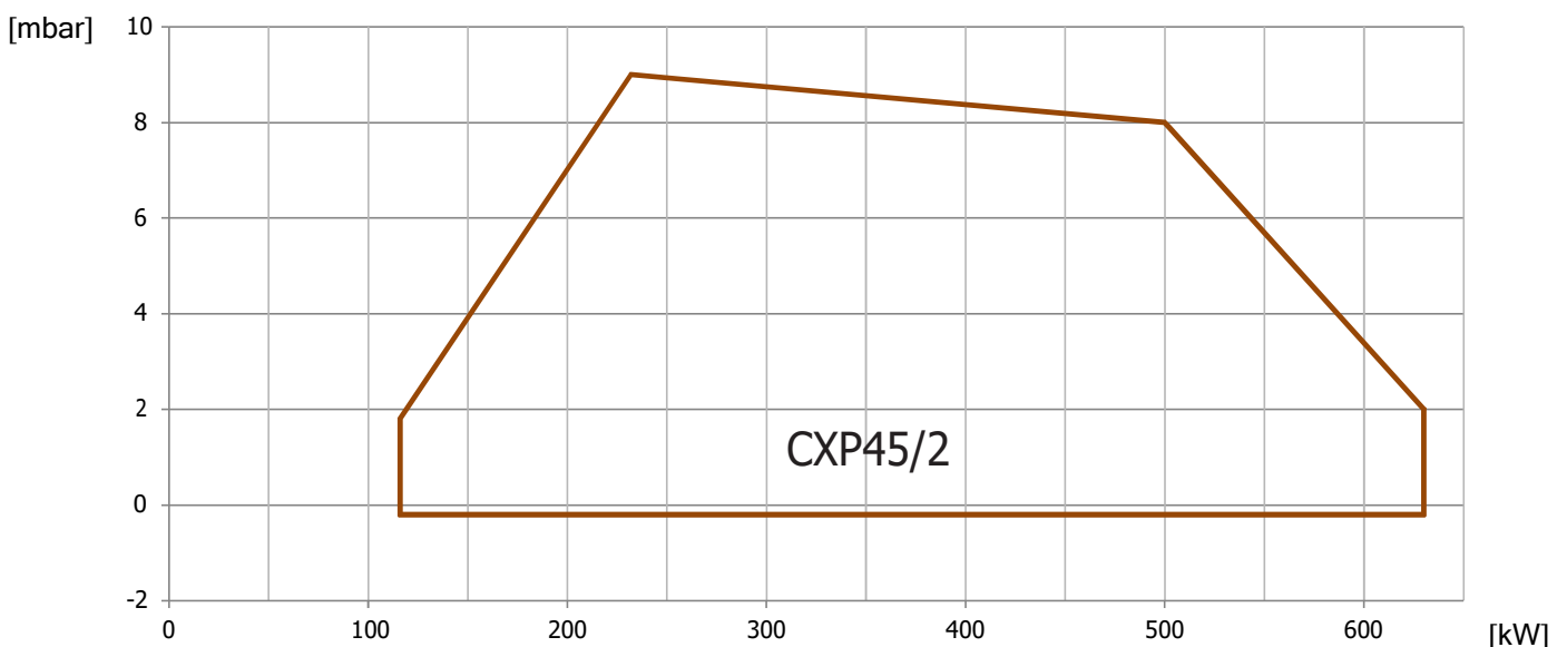
Fig. 2 X = Caudal Y = Presión en la cámara de combustión
