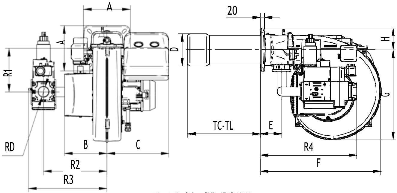
Fig. 3 Medidas CXP 45/2 MAX
